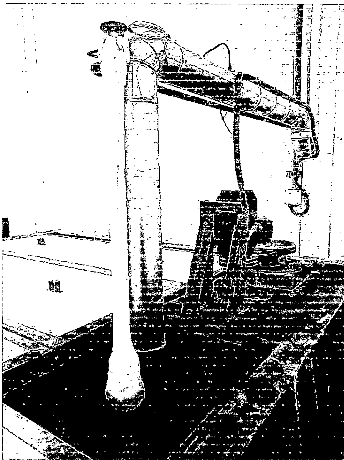
Fotografía N°13: Vista de pruebas de productor de hielo en bloques.
